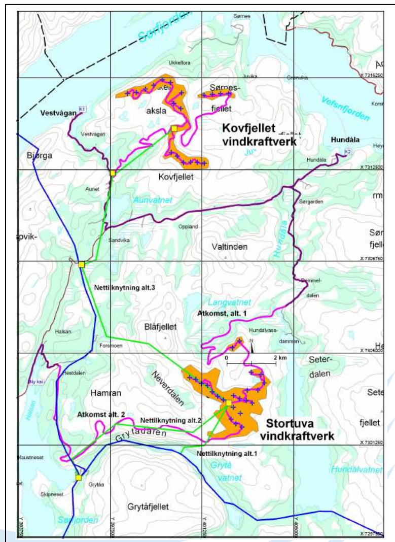
Figur 6: Innbyrdes plassering av Stortuva vindkraftverk og Kovfjellet vindkraftverk
